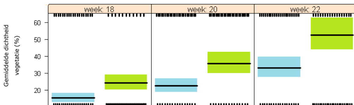
Figuur 18 De relatie tussen de gemiddelde dichtheid van de vegetatie op perceelsniveau en de aan- of afwezigheid van een greppel plas-dras, per week. Bovenstaande figuur is gebaseerd op het model met de laagste AICc-score (het beste model). Op de y-as staat de dichtheid van de vegetatie (in % bedekking). De horizontale zwarte streep toont de verwachte gemiddelde waarde op basis van het model. Aan de onder en bovenzijde van deze streep zijn de 95%-betrouwbaarheidsintervallen weergegeven. De linker (blauwe) balk toont de situatie op percelen met greppel plas-dras. De rechter (groene) balk toont de situatie op percelen zonder greppel plas-dras.
