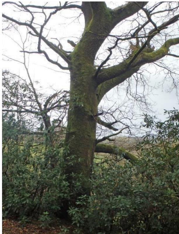
Fig. 35. Tree 3/20.
