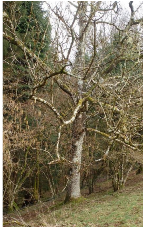
Fig. 29. Tree 3/3.
